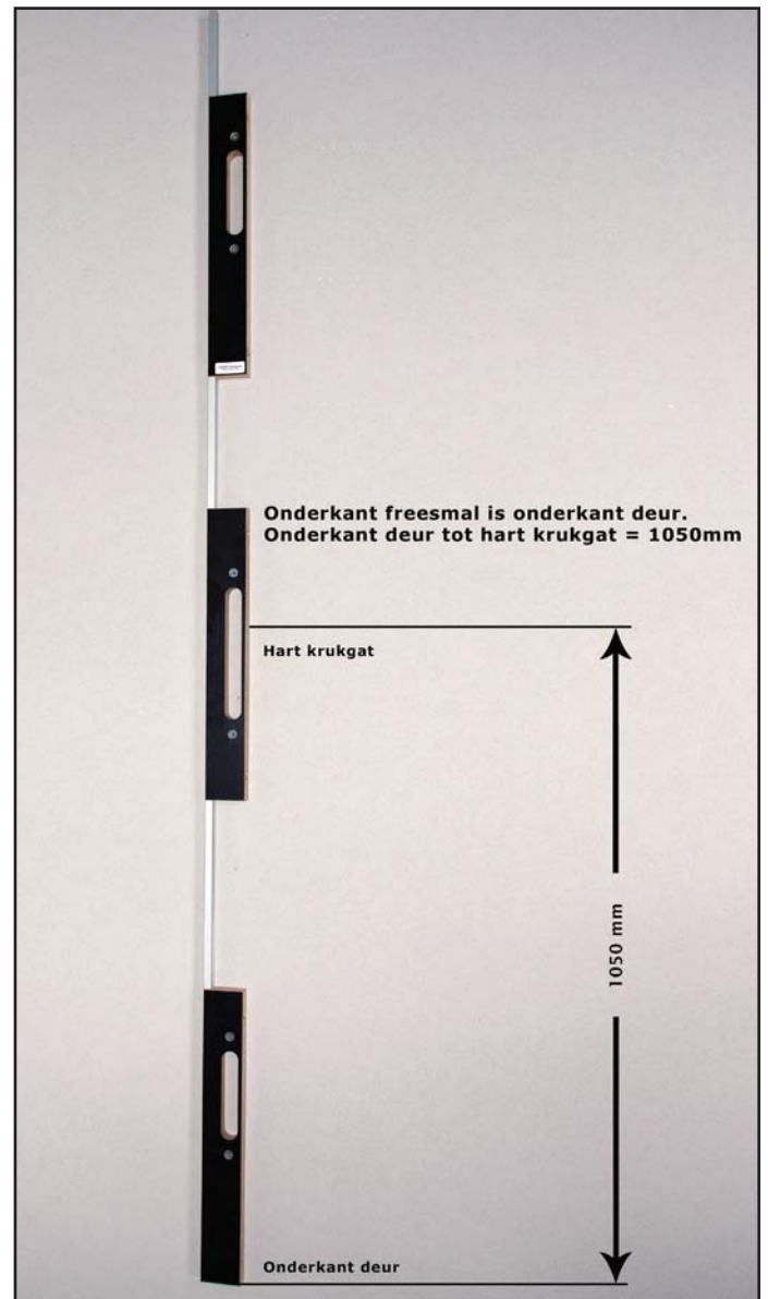
fig. 2 - Complete freesmal op strip (Lengte 2,12 meter)
